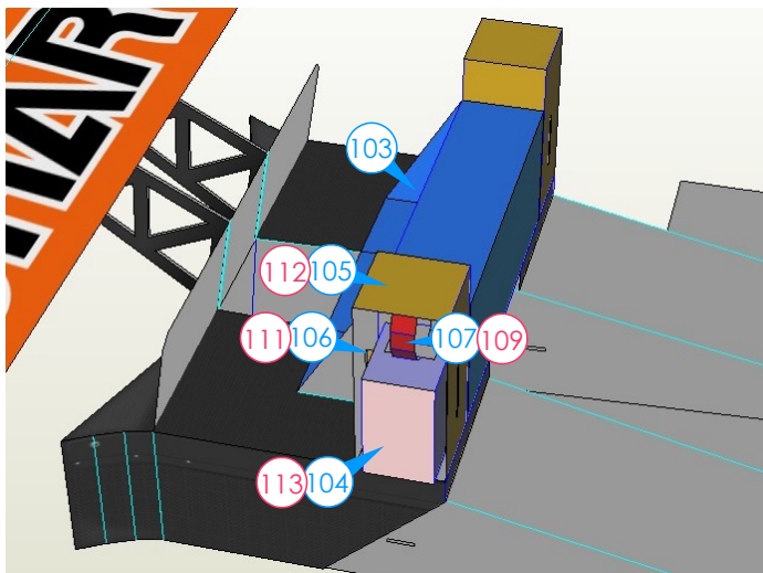
リアサスペンションの番号指定図
